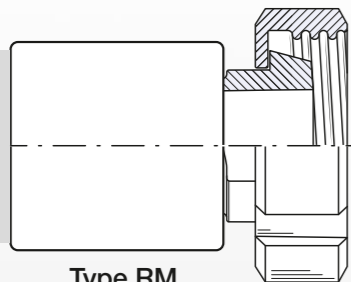
Type RM (Dairy Coupling, Female) DIN 11851
