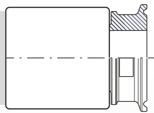
Type CF (Triclamp / Clamp Flange) DIN 32676
